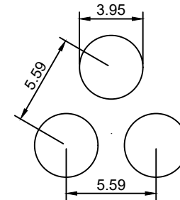
Detail 1:3
