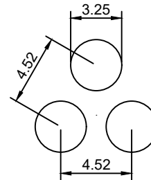
Detail 1:3
