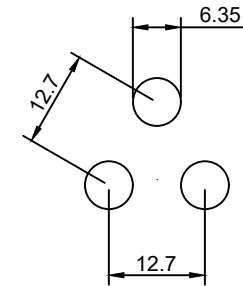
Detail 1:1
