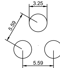
Detail 1:3
