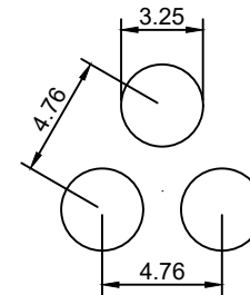
Detail 1:3
