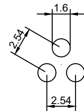
Detail 1:3
